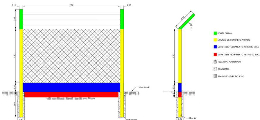
Figura 01 – Dimensões para instalação de cerca tipo alambrado.
